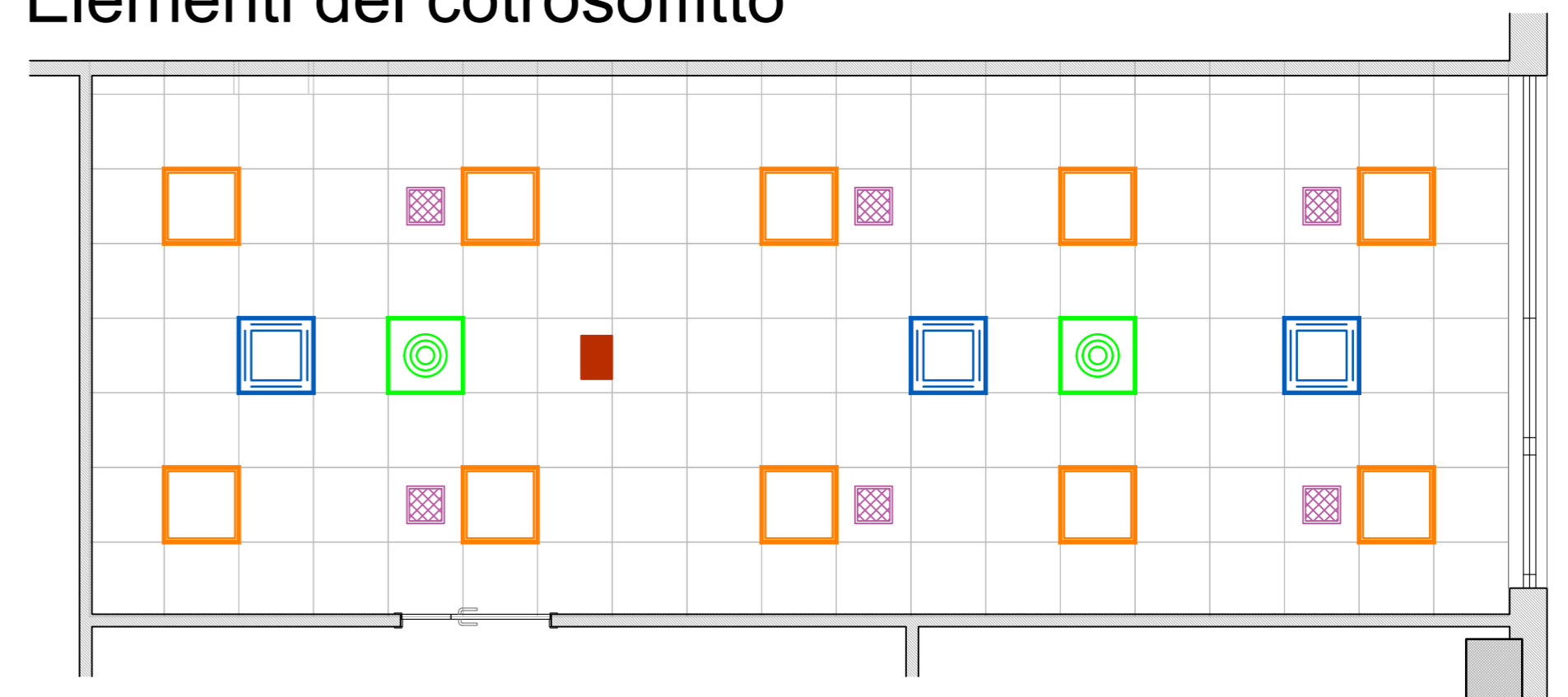
Elementi del cotrosoffitto
