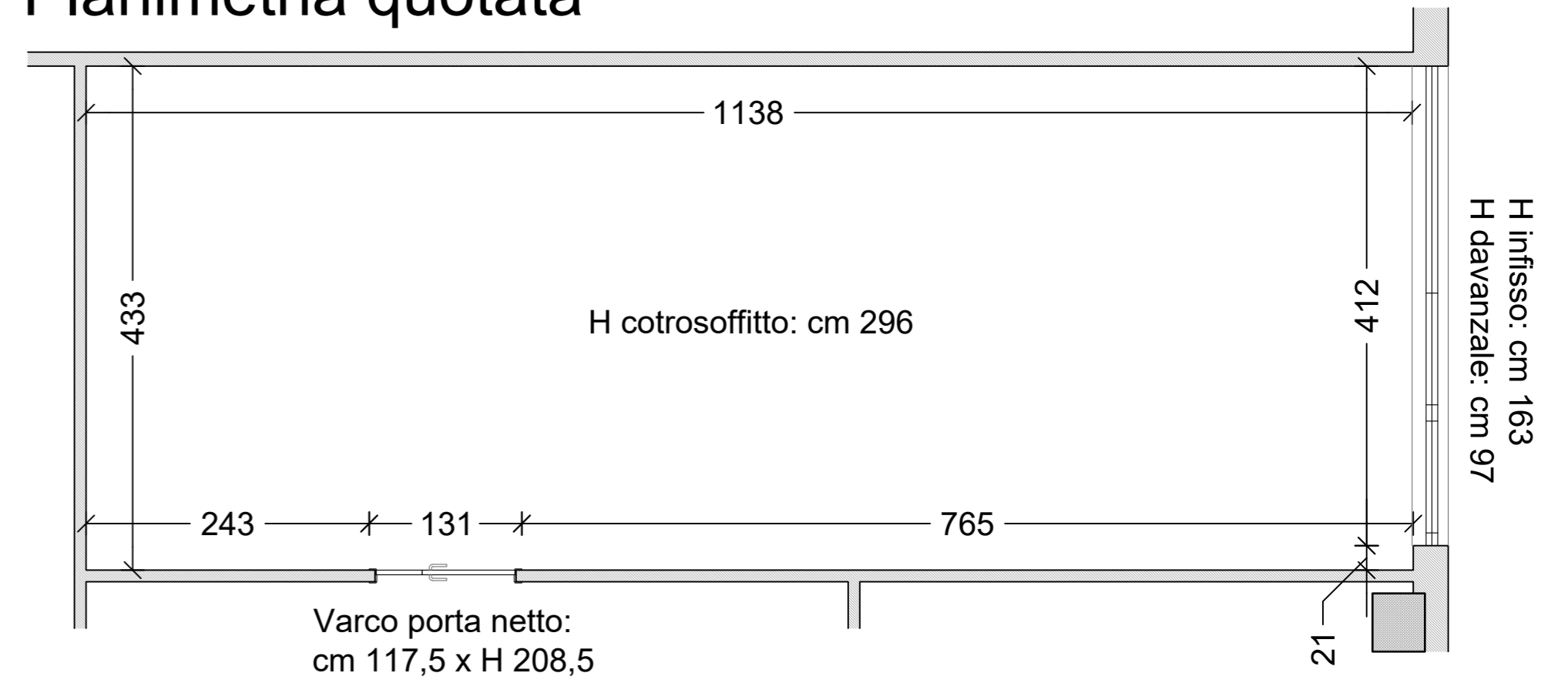
Planimetria quotata
